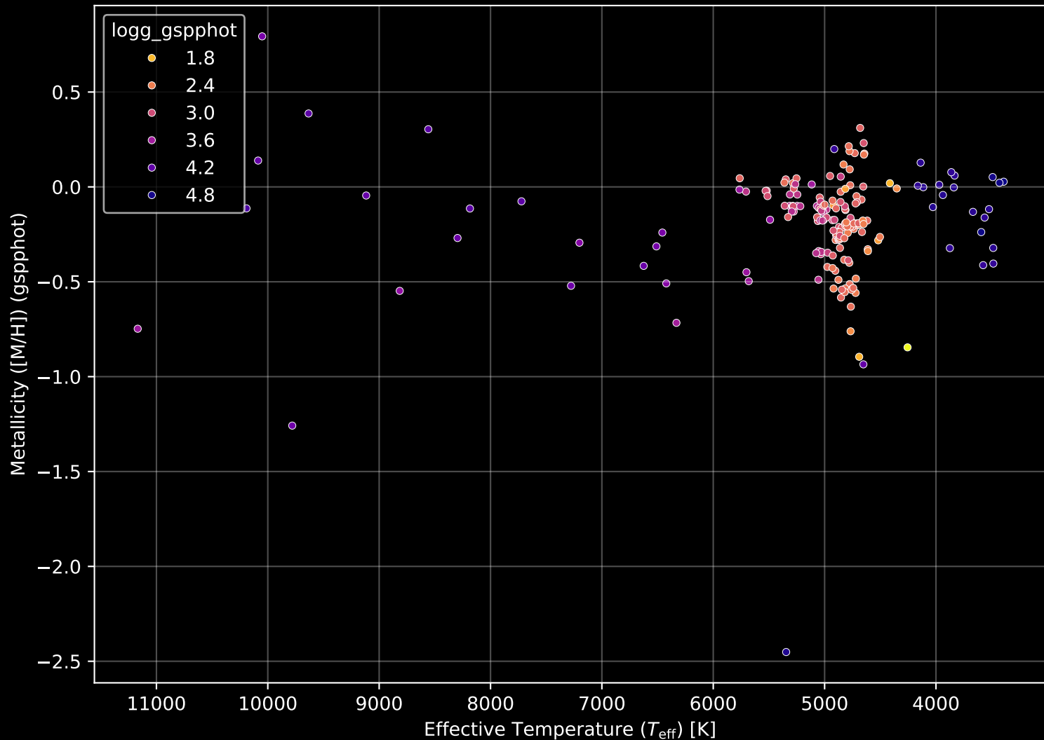
APOGEE DR17 Field: [NGC2420_btx] Stellar Population Parameters (n= 192)
